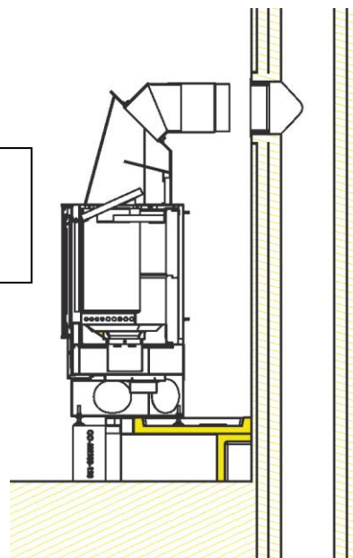
Obr. 10+11: Umístění krbové vložky do určené polohy
