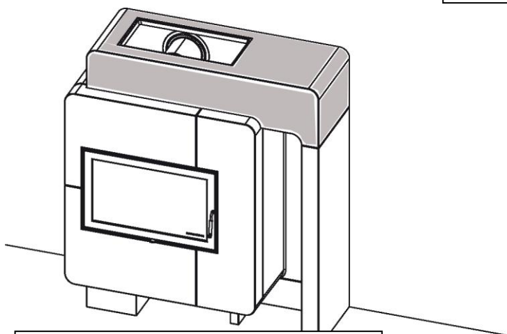
Obr. 27: Montáž stropního prvku
