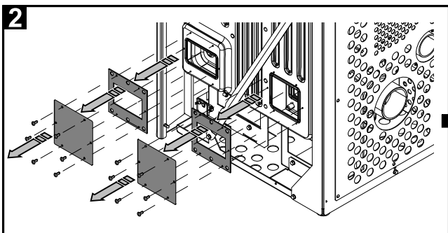
Rysunek 3a: Demontaż ściany bocznej (HSP 6 Rueda PGI)
