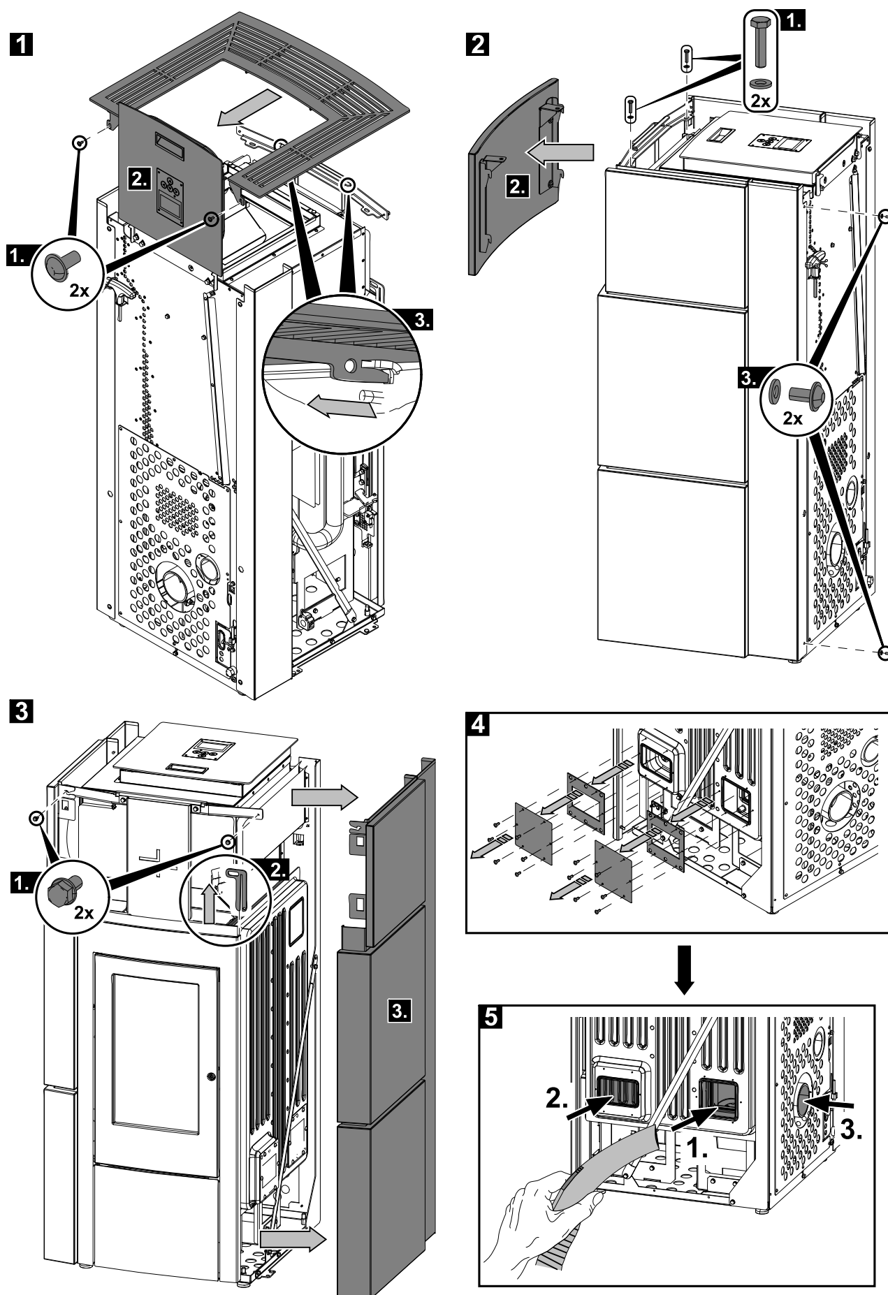
Rysunek 3c: Demontaż ściany bocznej (HSP 6 Rueda C PGI)
