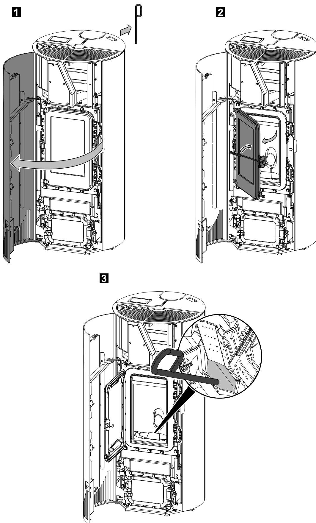
Obrázek 2: Čištění hořáku
