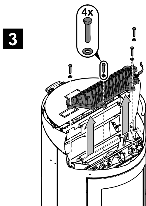
Obrázek 5: Čištění turbulátorem
