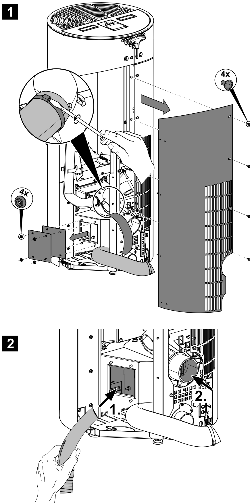
Obrázek 4: Demontáž boční stěny
