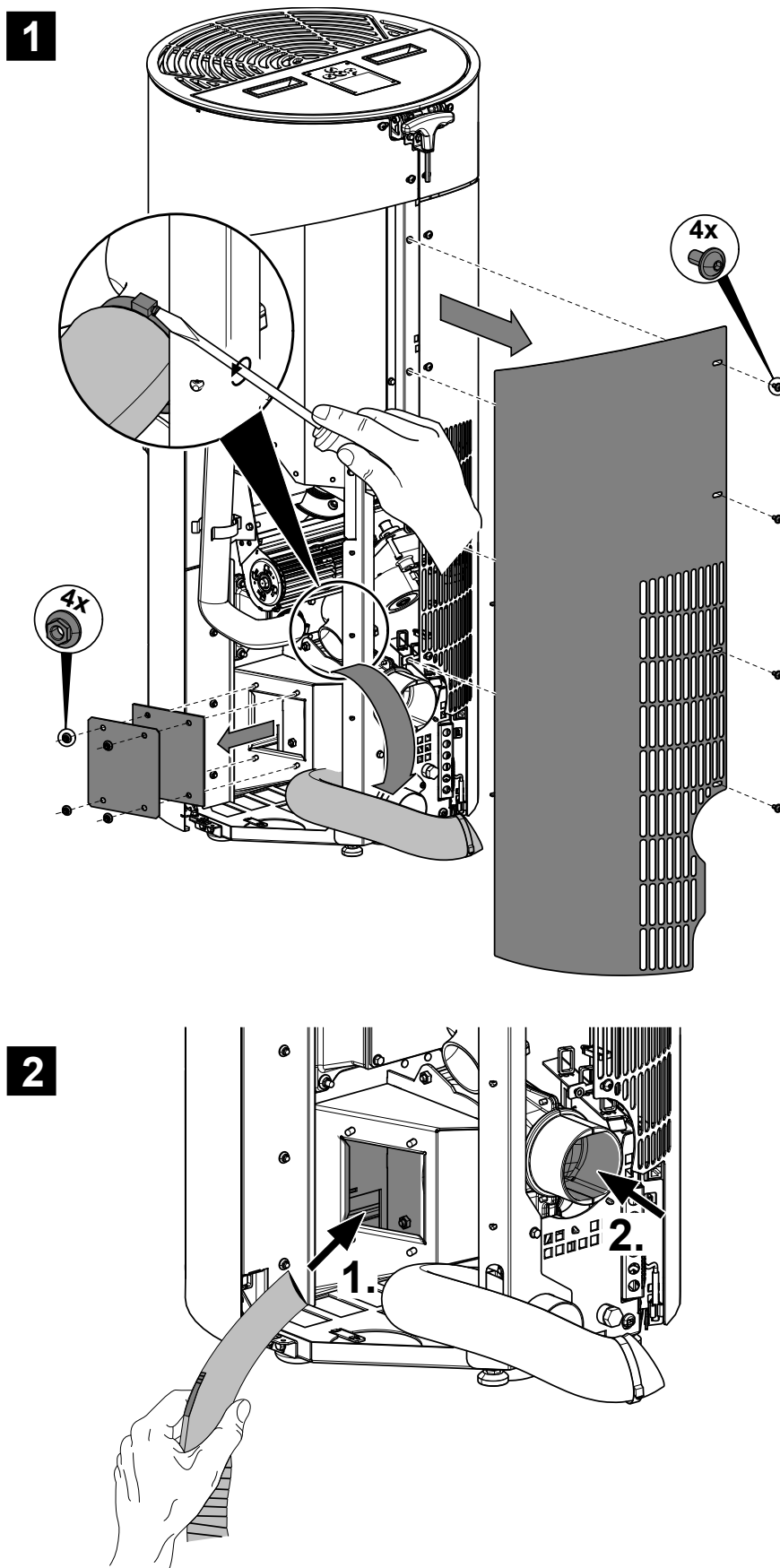
Rysunek 4: Demontaż ściany bocznej
