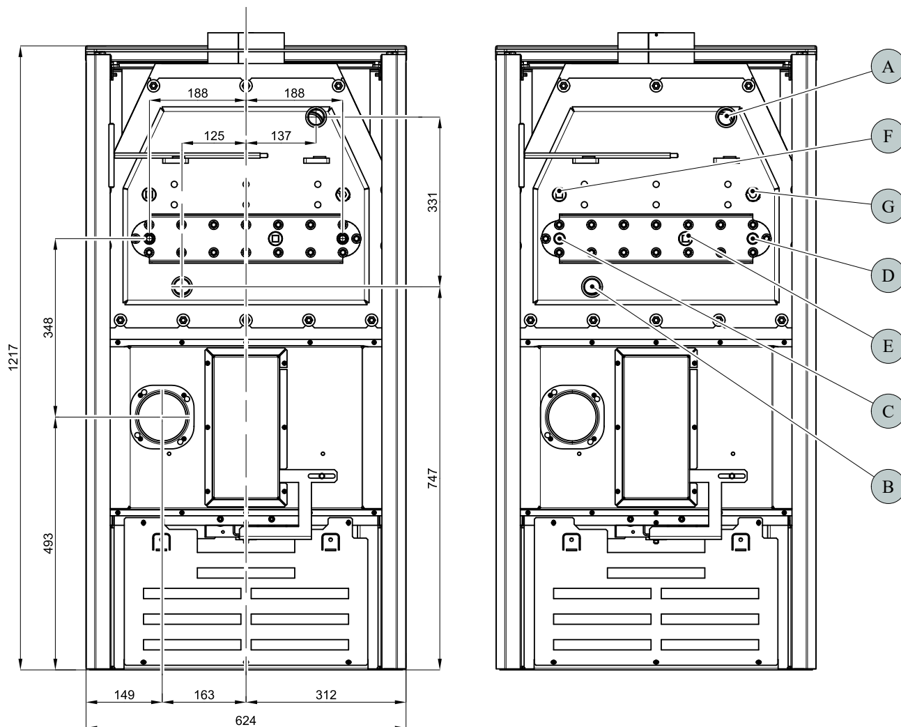
Rozmerová schéma
