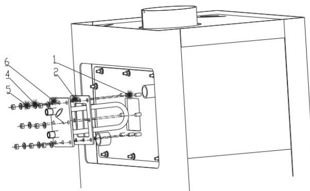
Montáž vychl. výmenníka
