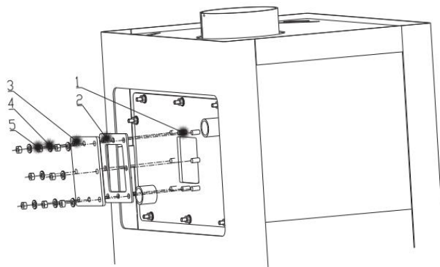
Demontáž záslepky
