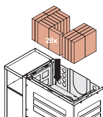
AKUMULAČNÍ SADA AXON 92 kg (není součástí) 0433120000099
