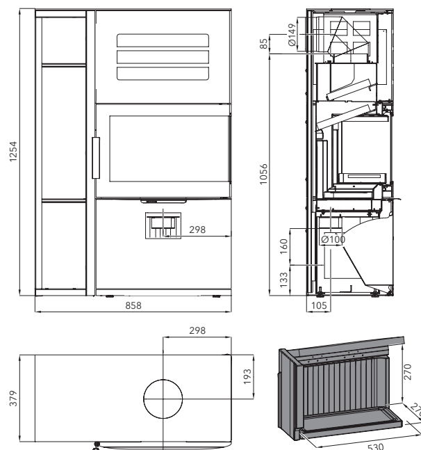
AKUMULAČNÍ SADA AXON 92 kg (není součástí) 0433120000099
