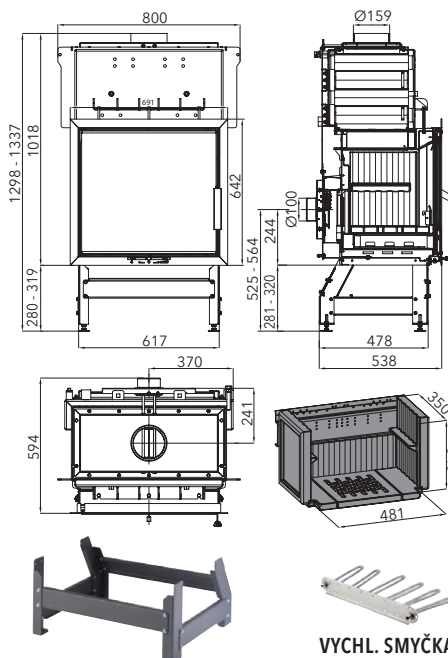
MONTÁŽNÍ SADA VESUVIO II (není součástí) 0619018151300
