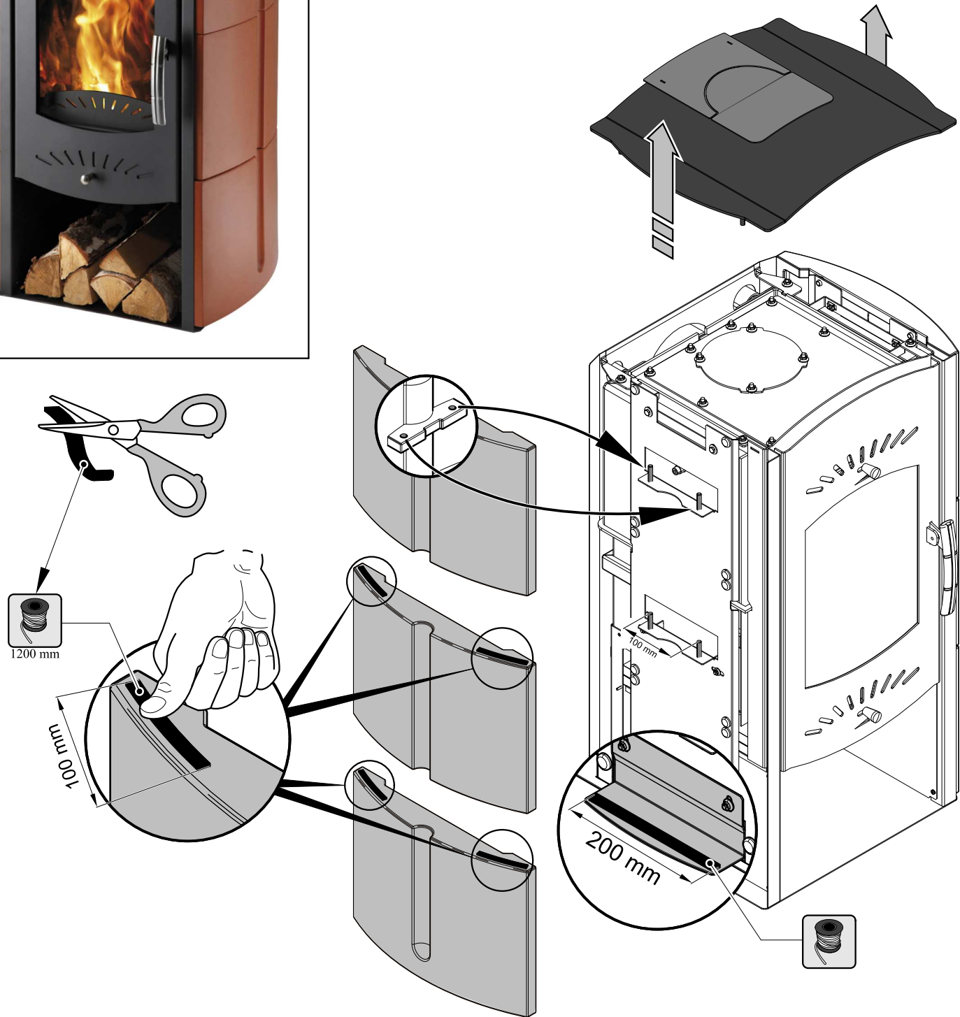
Montáž vymezovací šňůry kachlí
