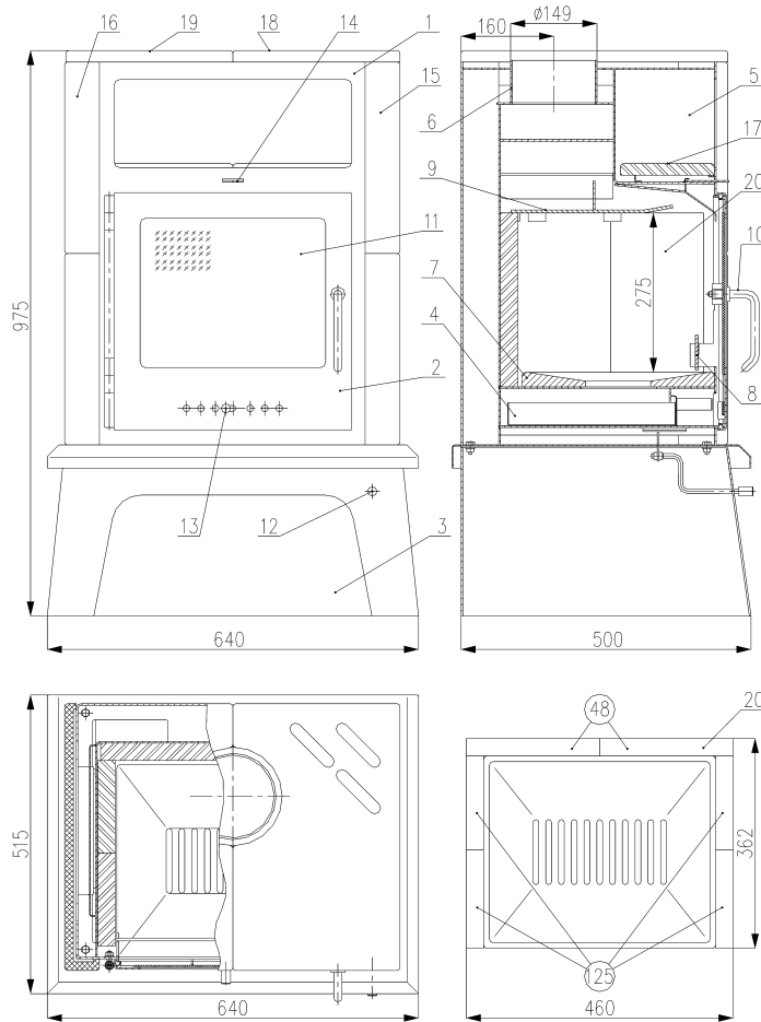
Šamotová vyzdívka
